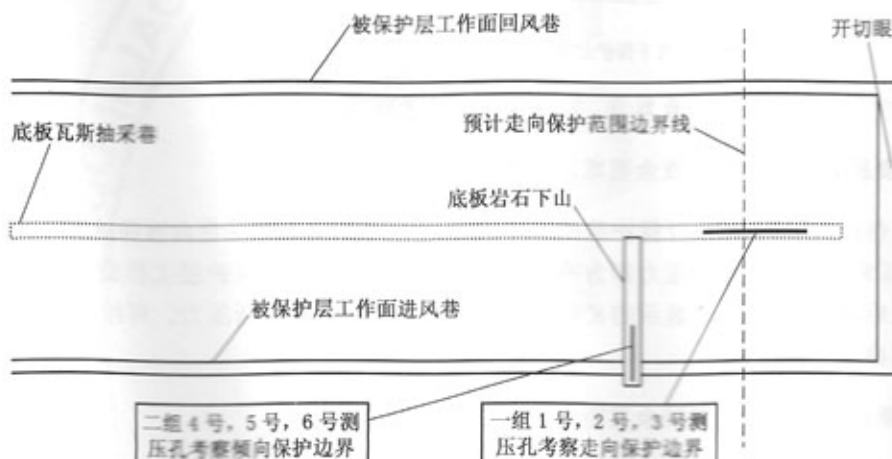
图 B.1 走向及倾向保护范围考察方案示意图
