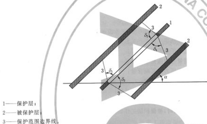
图 A.1 保护层工作面沿倾斜方向的保护范围
