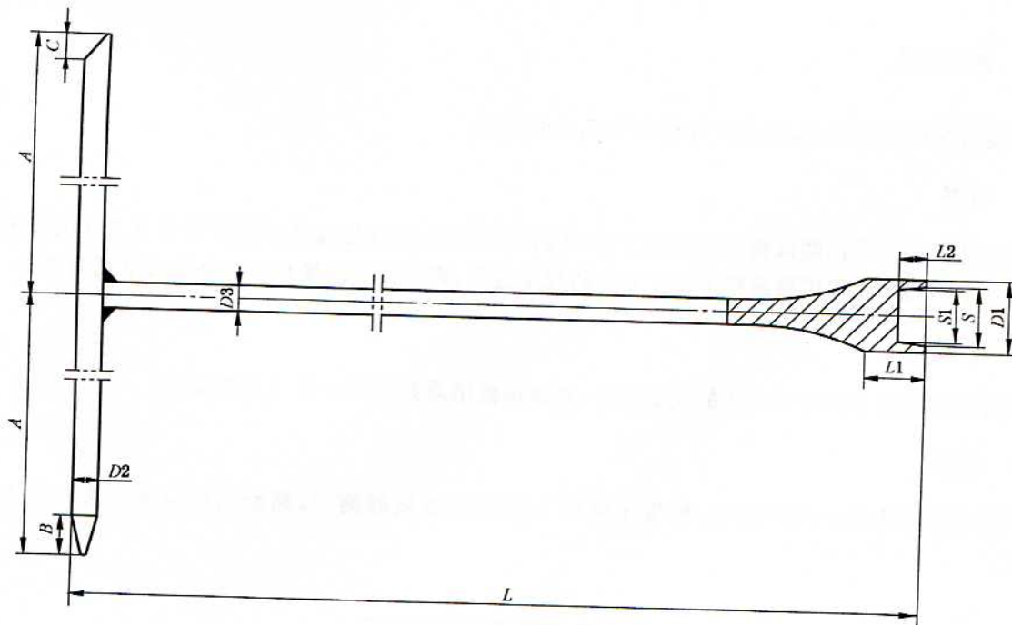
图 B.2 地下消火栓扳手
