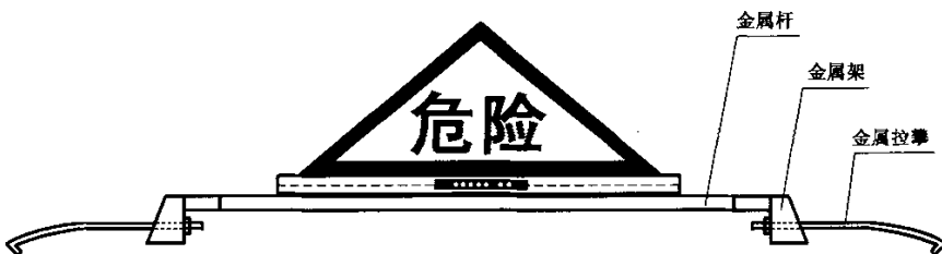
图 2 B 型标志灯
