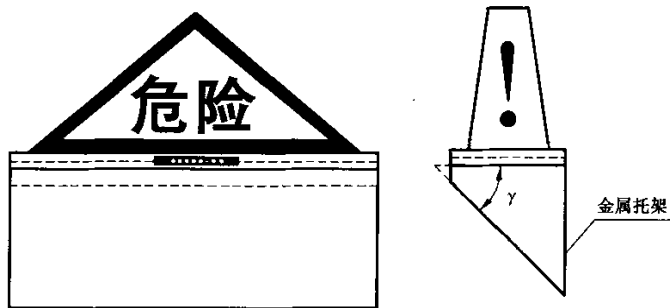
图 3 C 型标志灯
