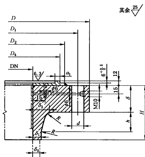
图6 衬环棒密封面(C-T)
