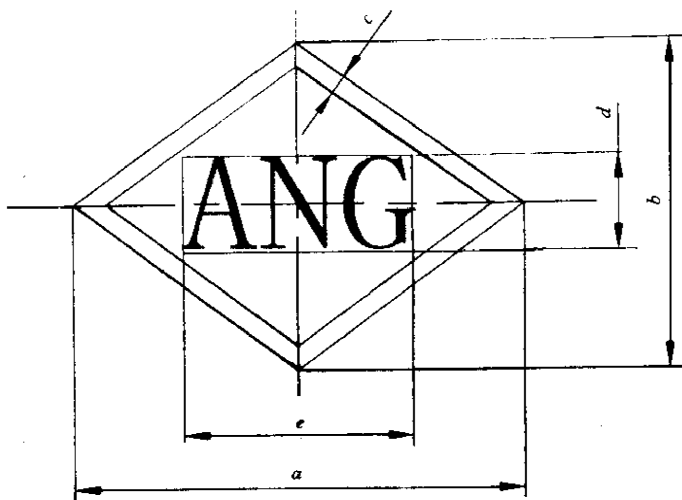
图 3 吸附天然气汽车标志图形
