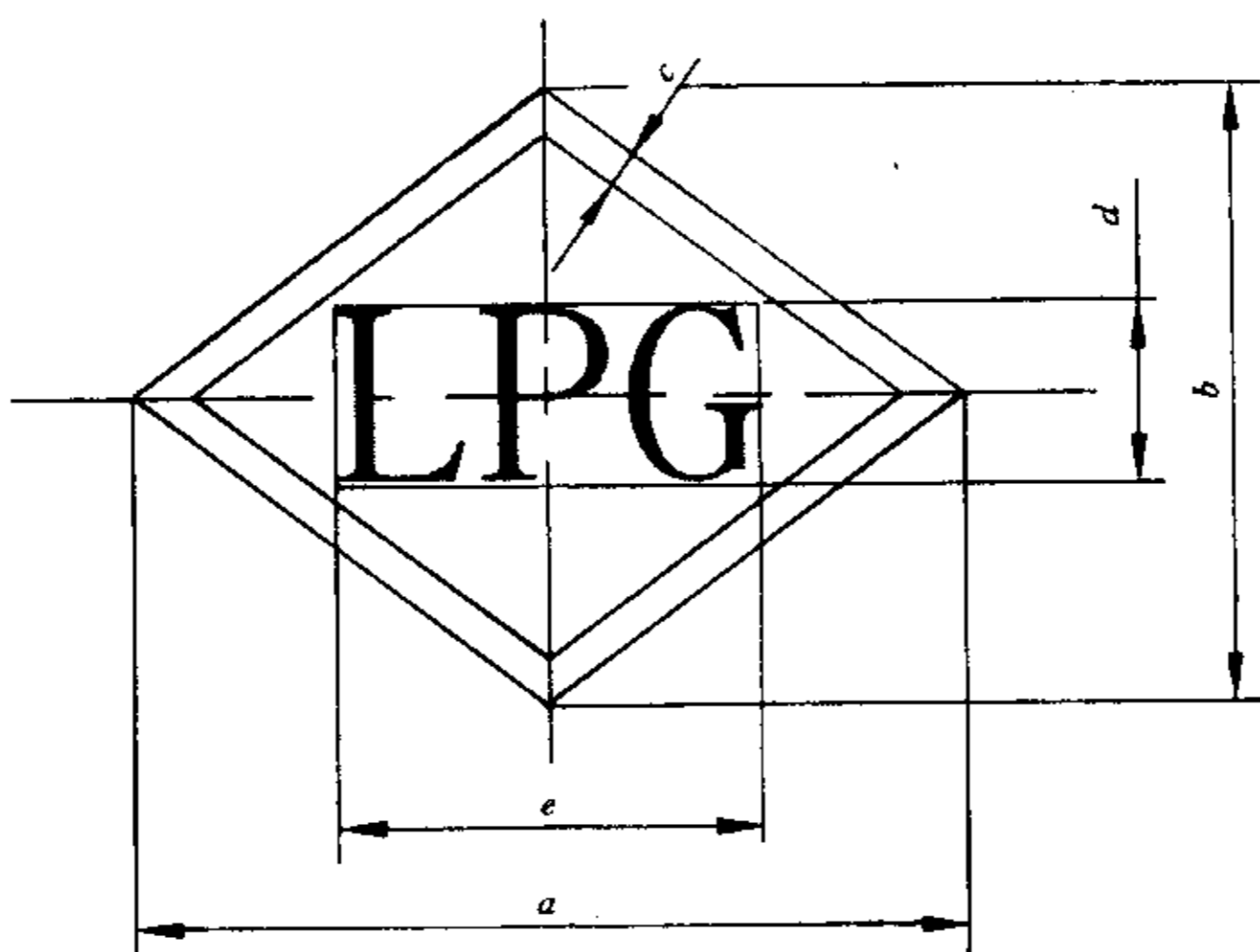
图 4 液化石油气汽车标志图形
