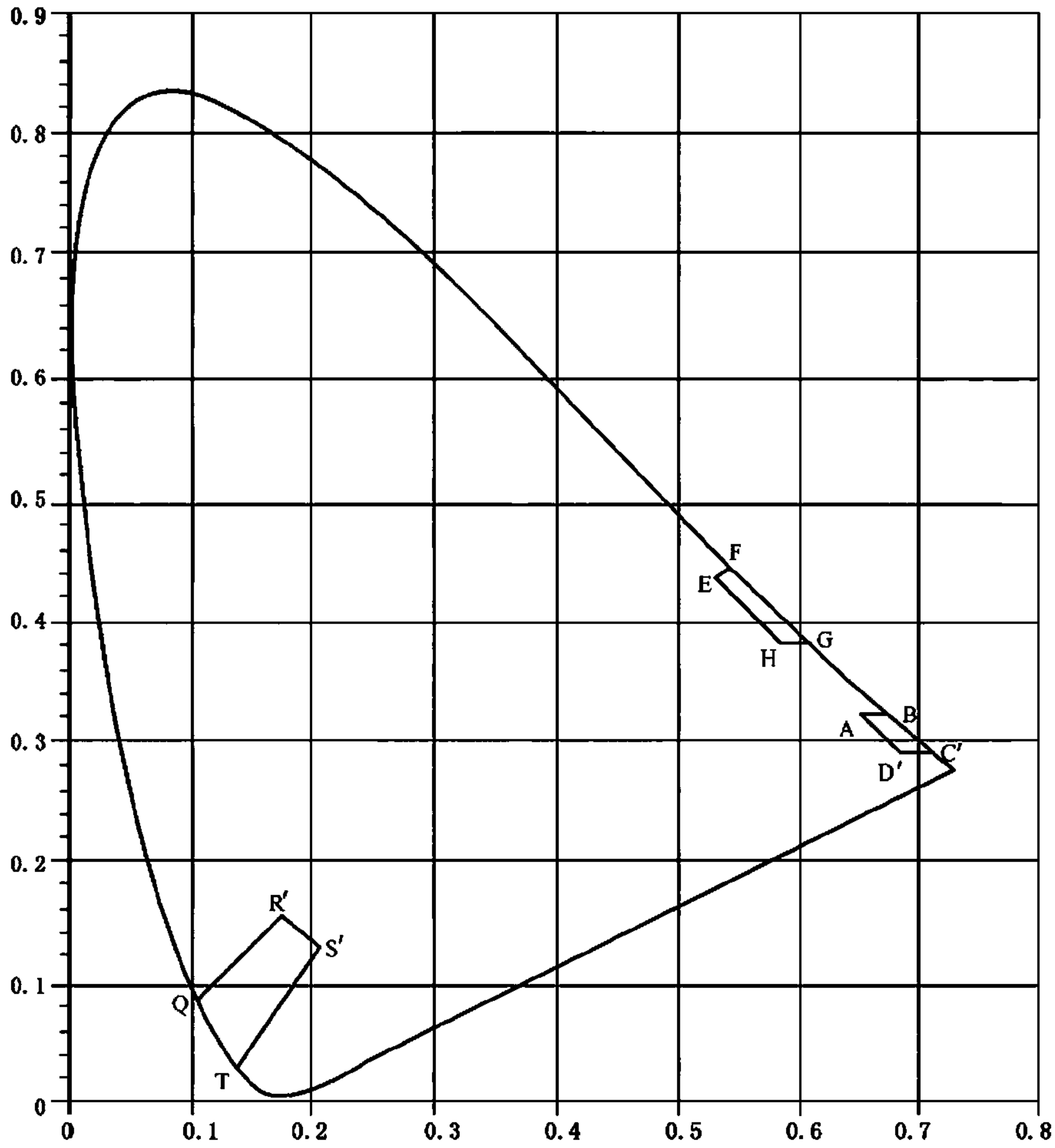
图 A.1 标志灯具灯光颜色色品图
