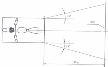
图 A.2 后视白光的不可见度
