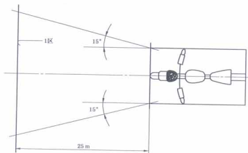
图 A.1 前视红光的不可见度
