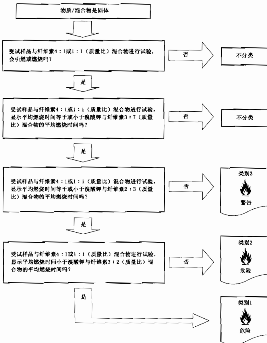
图 1 氧化性固体判定流程
