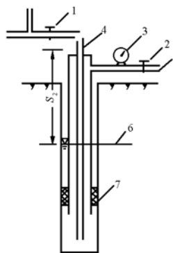
图 A2 回水管上安设压力表示意图
