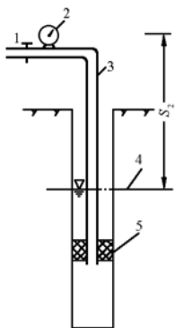
图 A1 进水管上安设压力表示意图
