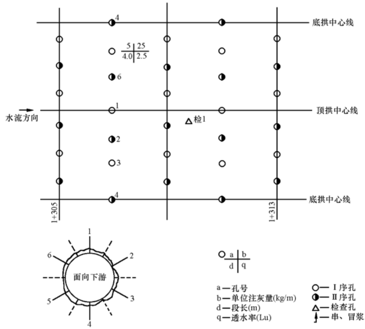
工程隧洞固结灌浆成果展示图
