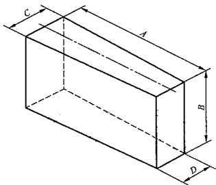
图 4 竖厚楔形砖
